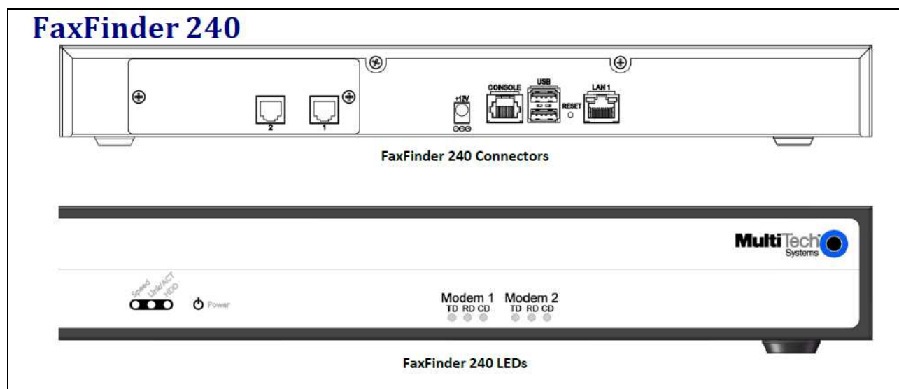
Fig.4 Connessioni
