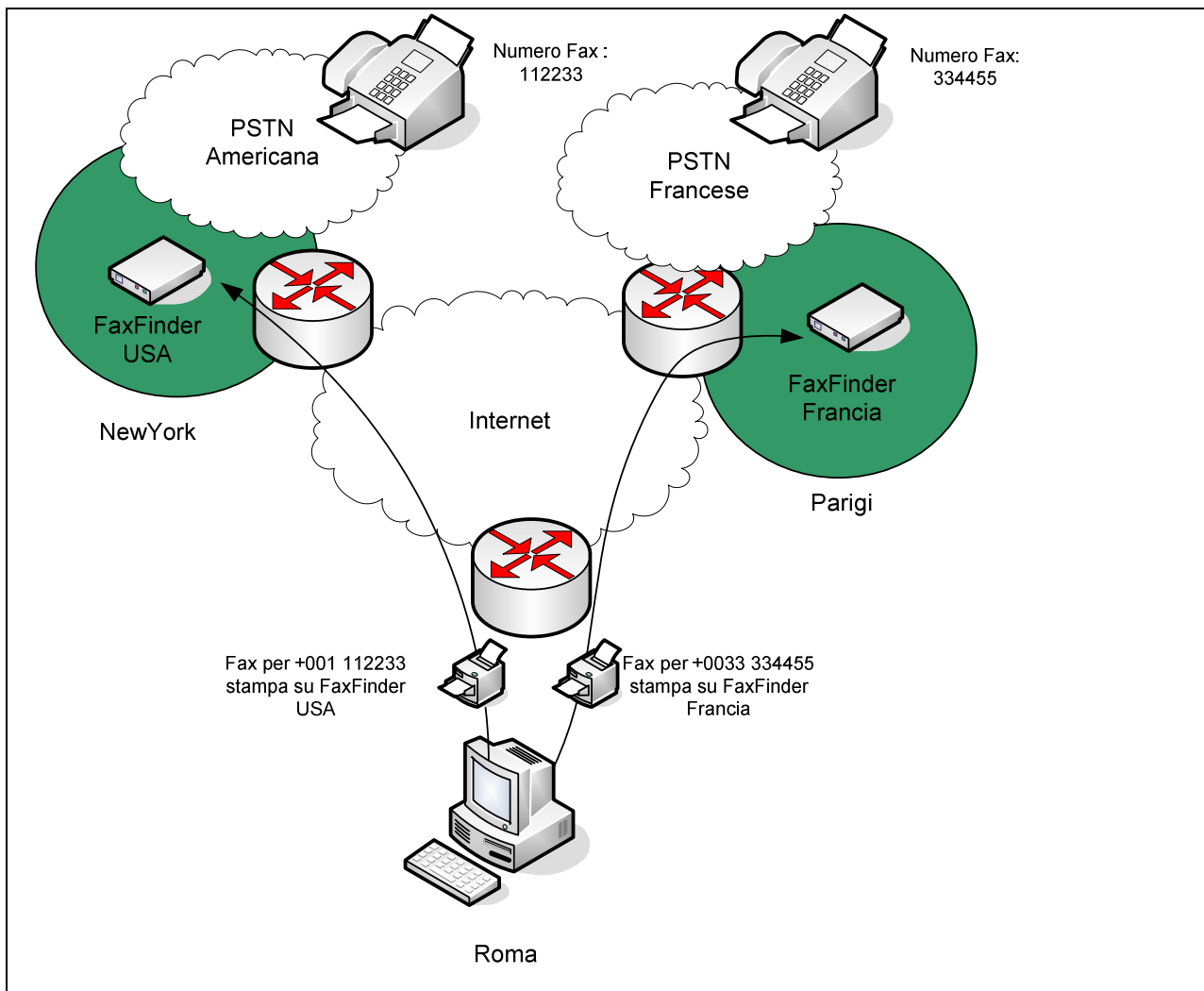
Fig. 3 Esempio applicativo
