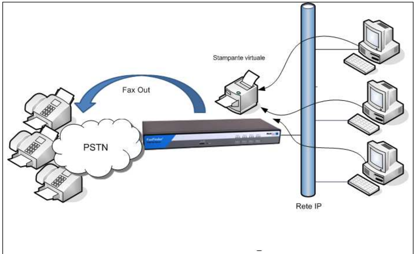
Fig.2 – Trasmissione di fax
